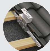
Läktfäste med fäste för falsad panna.
