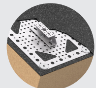
Tätplåt OPTI med konsol för skena (för papp eller duk).
