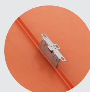
Falsfäste till bandtäckning och clicktak.
